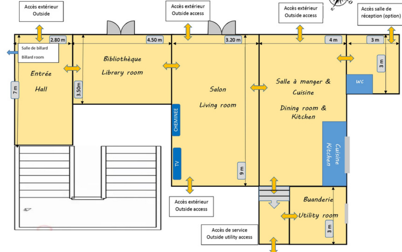
GITE DOMAINE GAVOTY - PLAN 2ème ETAGE / SECOND FLOOR
